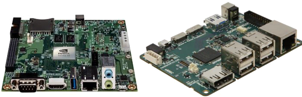
< 그림 IV-18 > Nvidia Jetson TK1 & Odroid XU3
